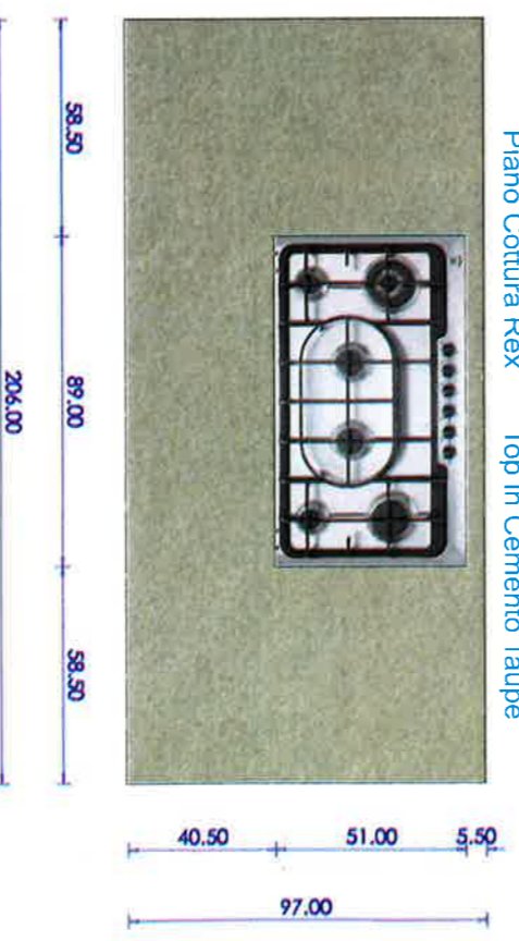
PROSPETTO
