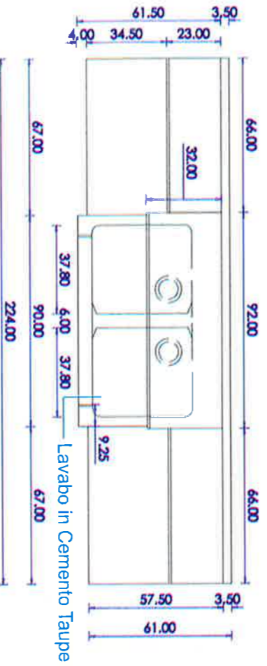
PIANTA
