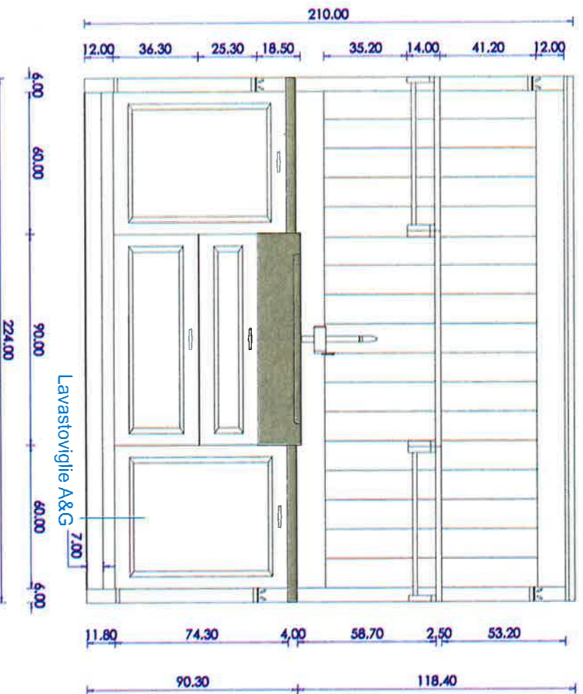
PROSPETTO
